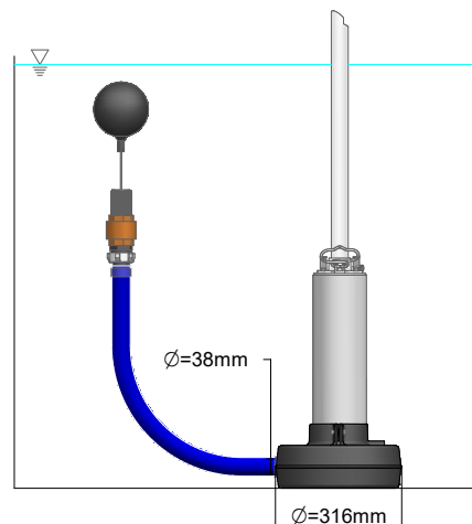
Exemple d'installation d'un socle d'aspiration en surface
